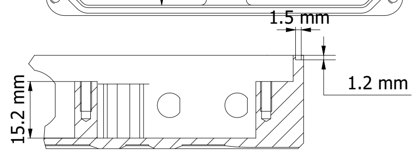
A-A ( 1 : 1 )
